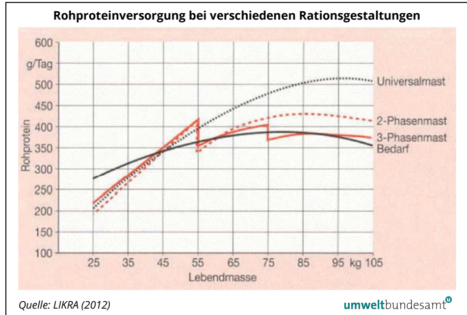
Abbildung 2: Rohproteinversorgung bei verschiedenen Rati- onsgestaltungen (Schweinemast).
