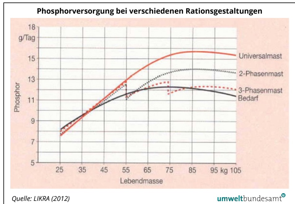
Abbildung 3: Phosphorversorgung bei verschiedenen Rations- gestaltungen (Schweinemast).
